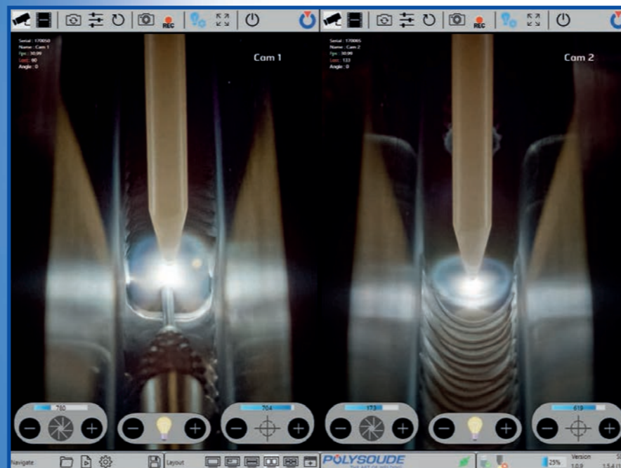
Наблюдение за сварочным процессом с нескольких камер
